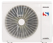
Buitenunit Marvin SOH-09BIM 2,7 kW 220/240-1-50Hz warmtepomp inverter R32
