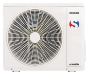
Buitenunit Marvin SOH-18BIM 5,3 kW 220/240-1-50Hz warmtepomp inverter R32
